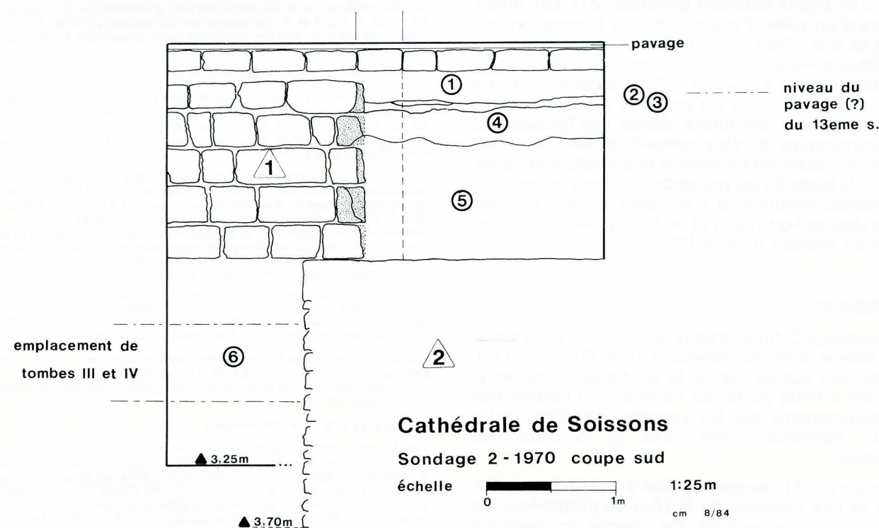
Fig. 5 : Coupe sud du sondage 2.
