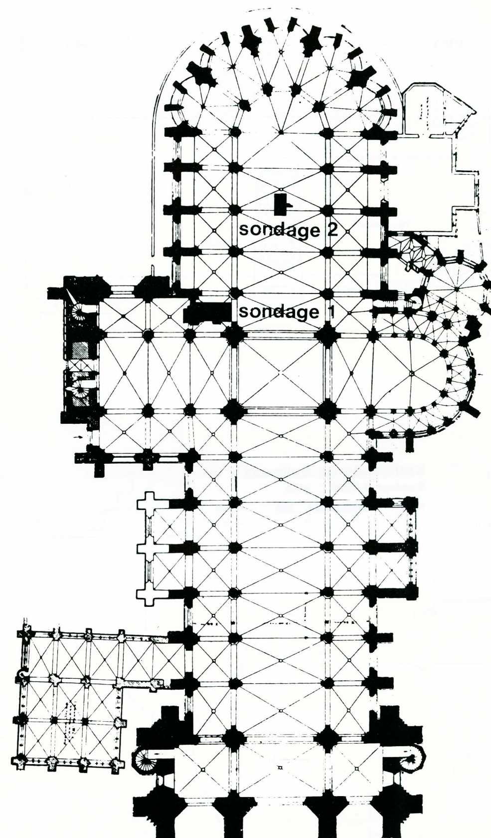
Fig. 1 : Plan de la cathédrale de Soissons d'après Brunet. Emplacement des sondages de 1970.
